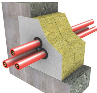
Intumex KH21 Brandschutz-Kabelhülse
