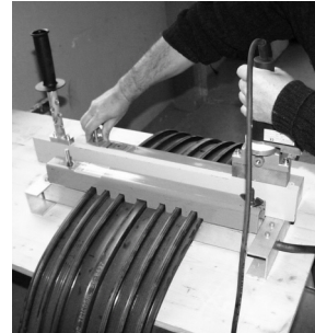
Saldatura in atelier e in cantiere.
